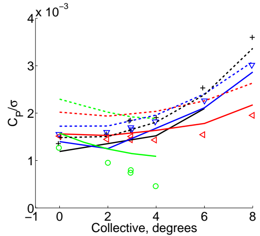
(d) Power coefficient, C_P/\sigma .
