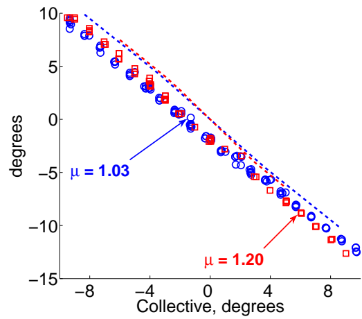
(d) \theta_{1S}, \mu > 0.825 .
